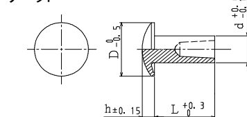
トラス(T) 材質:PB
