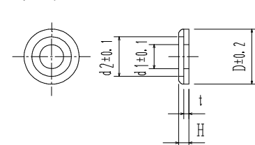
ワッシャー
