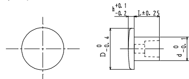
平頭(K) 材質:PC
